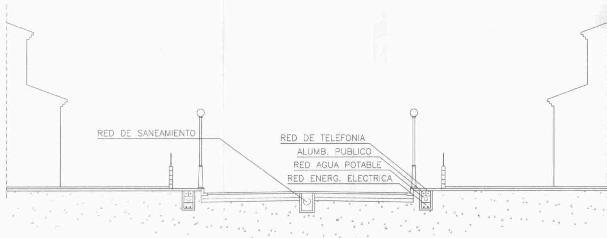
SECCION TIPO DE VIAES ESCALA 1:100
