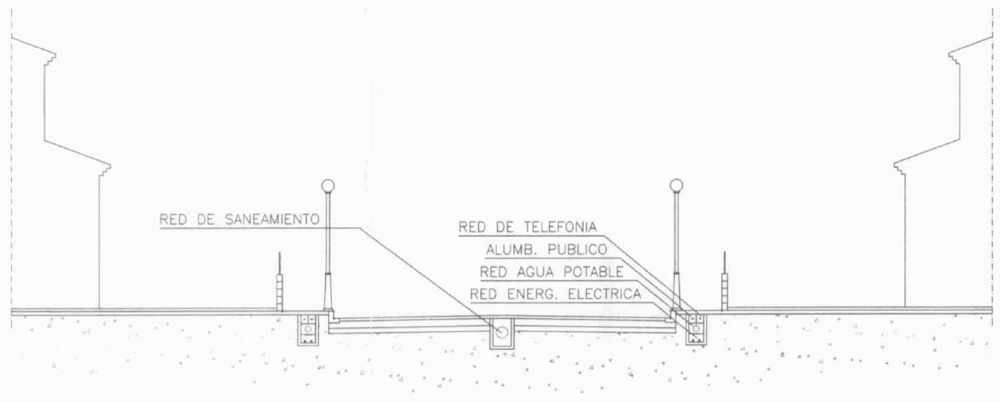
SECCION TIPO DE VIALES ESCALA 1:100
